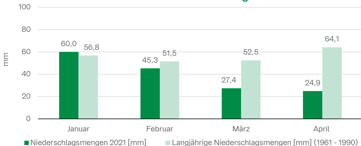
Monatliche Niederschläge
