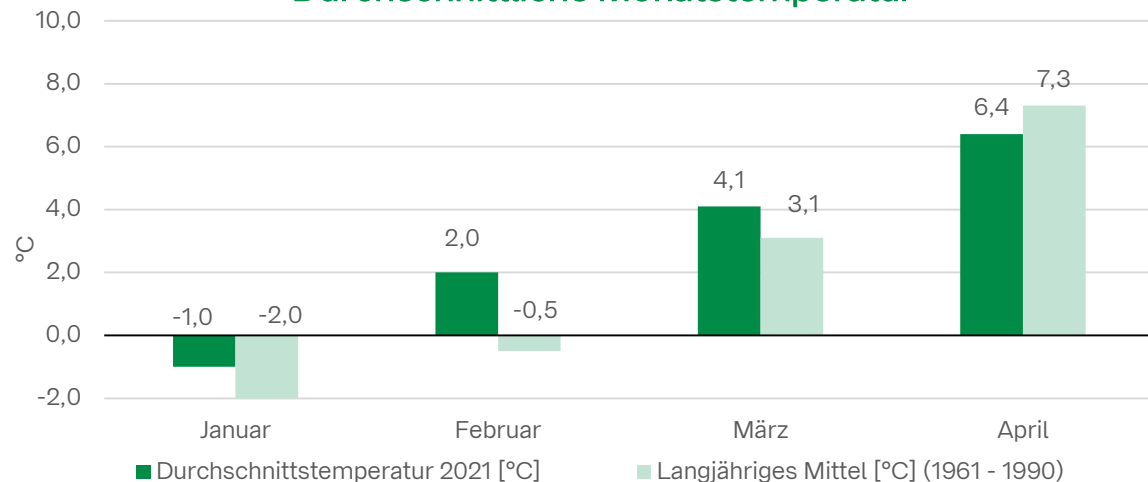
Durchschnittliche Monatstemperatur
