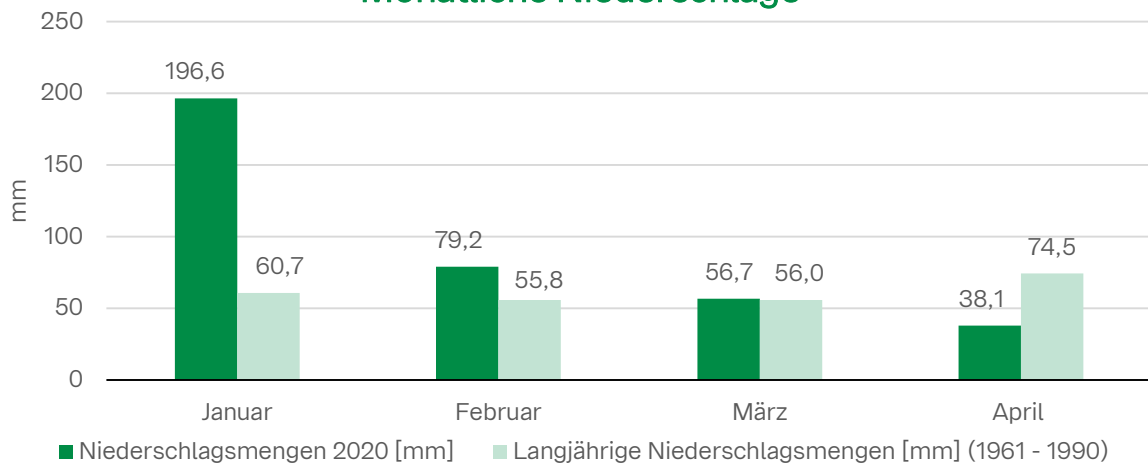
Monatliche Niederschläge
