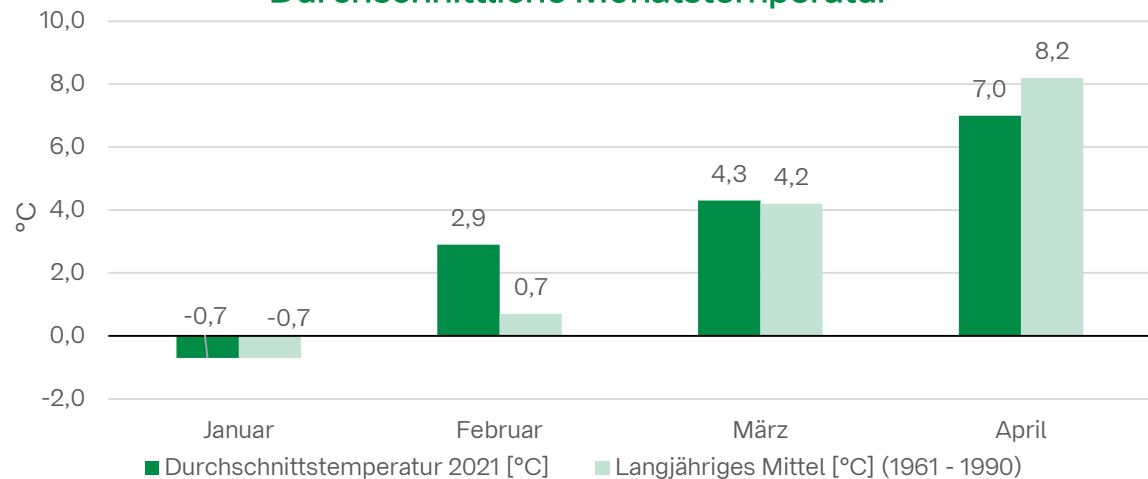
Durchschnittliche Monatstemperatur
