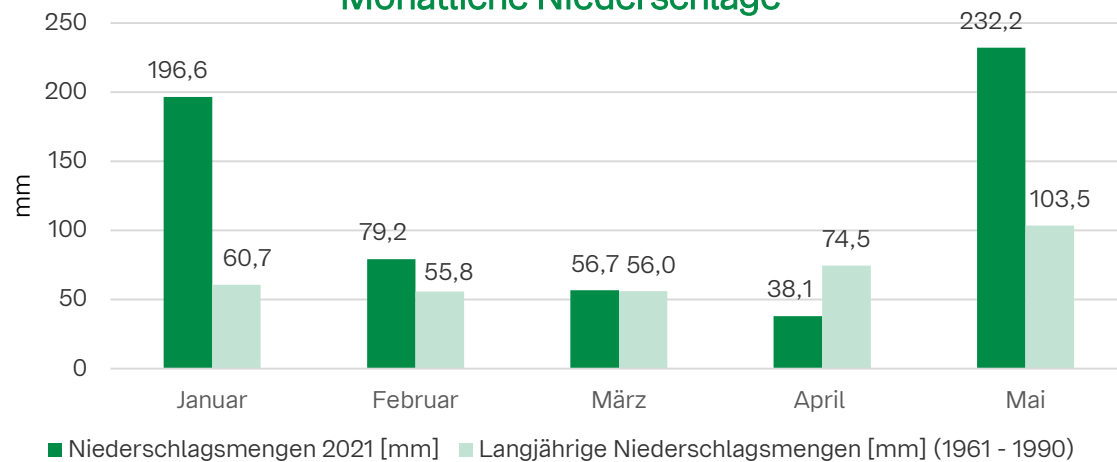
Monatliche Niederschläge
