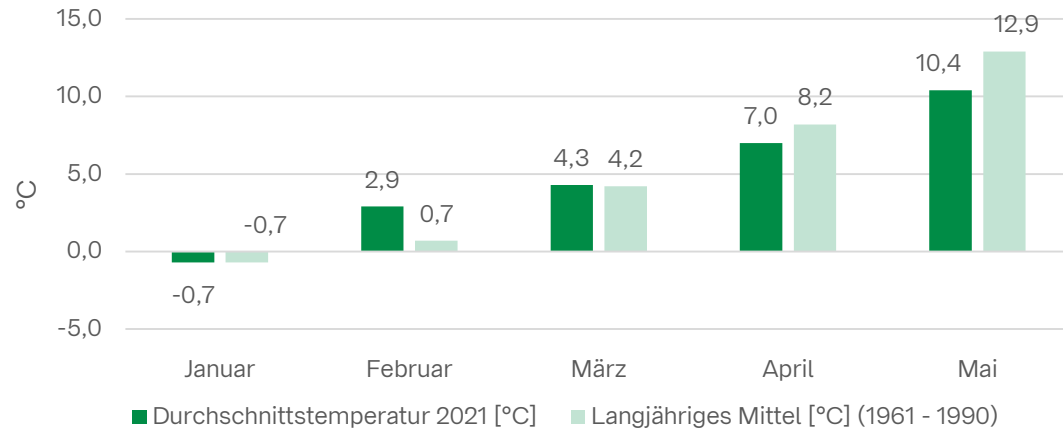
Durchschnittliche Monatstemperatur
